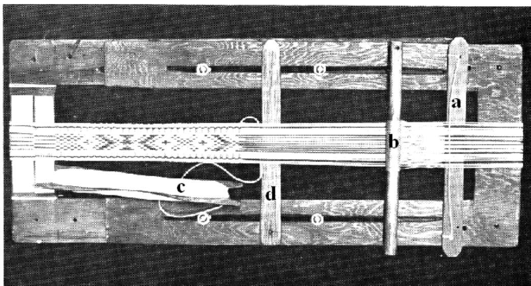
Rėmelis juostoms austi: a - skala b - nytelės c - šaudyklė d - medinis peilis
